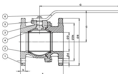
DN65-DN150
